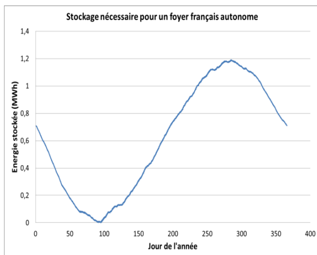
Evolution du stockage à partir de 3 kW c de panneaux photovoltaïques pour un ménage.
